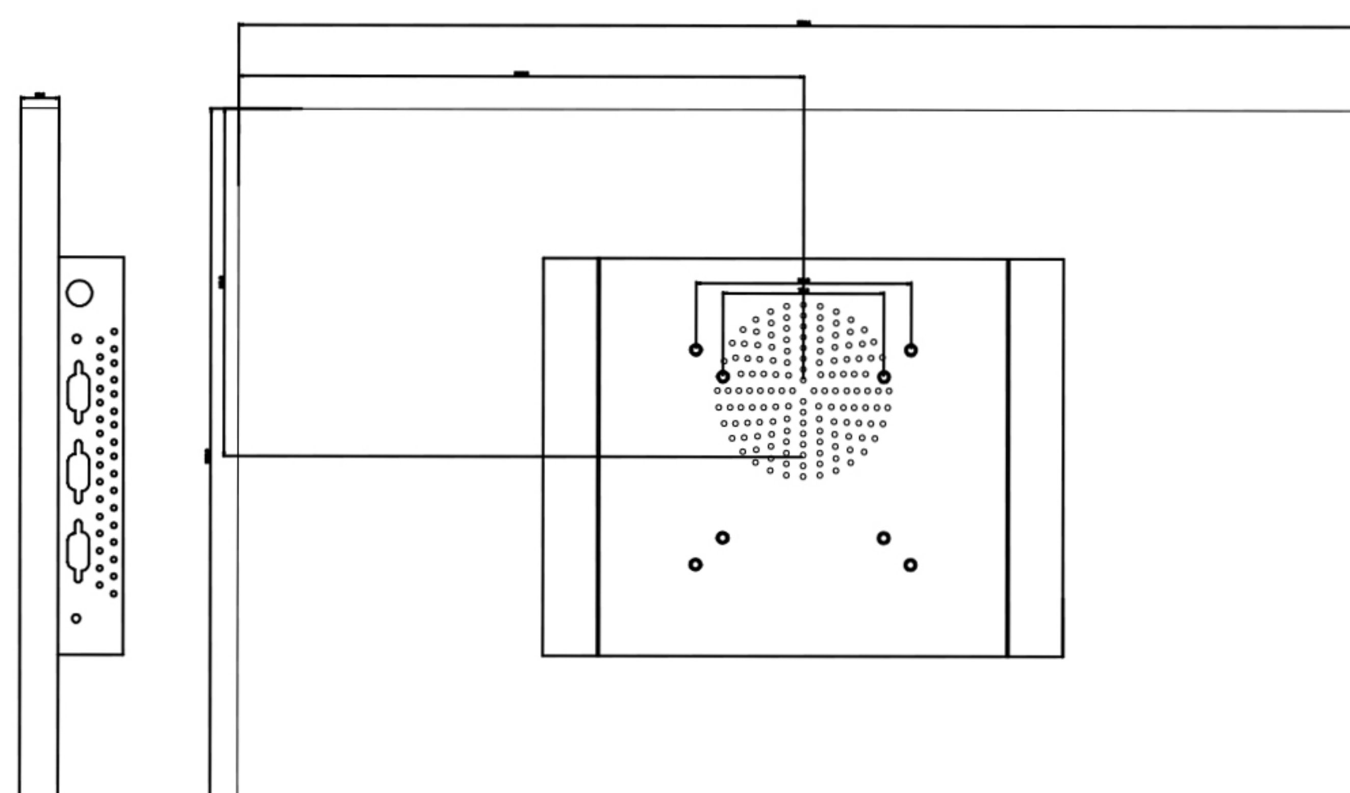
壁挂尺寸: 100*100 75*75
